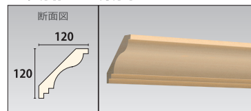
① 天井廻り縁直材 サンメント 品番：A470 サイズ（mm）：120（H）×120（D）× 3.650（L）
